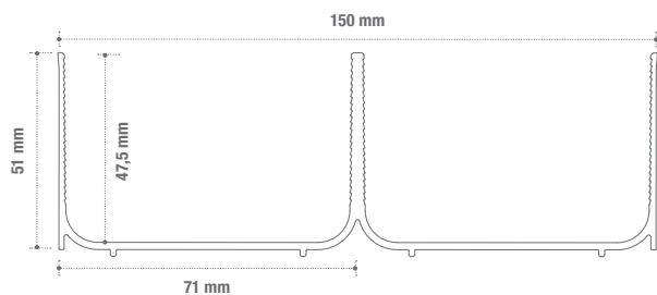
PROFILO PORTAPOSATE DOPPIO IN ALLUMINIO DOUBLE DRAWER DIVIDER IN ALUMINIUM
