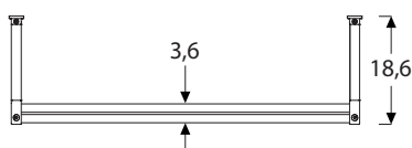
VISTA SUPERIORE TOP VIEW
