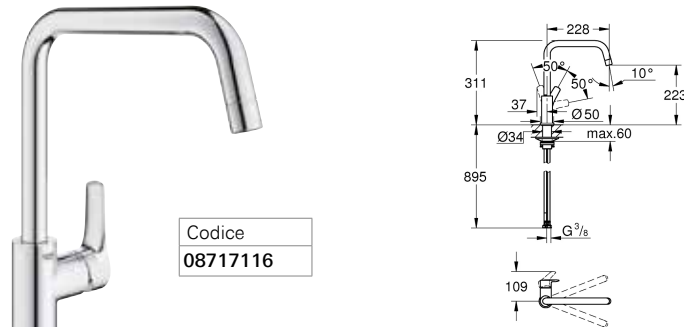
Eurosmart | bocca alta sottofinestra
