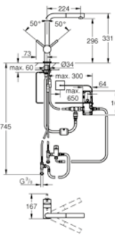
Minta Touch | bocca L | doccetta estraibile
