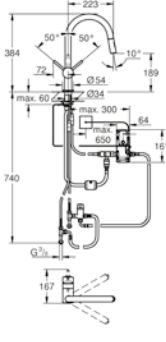
Minta Touch | bocca C | doccetta estraibile
