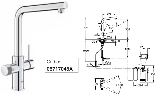
New Minta | bocca L
