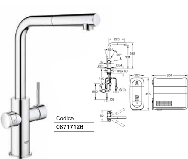
Blue Home | bocca L | doccetta estraibile
