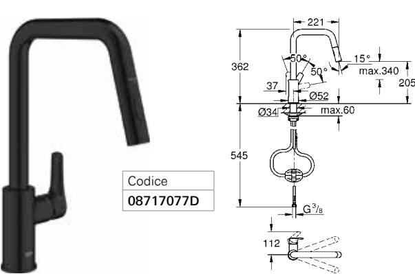
Eurosmart | bocca alta | doccetta estraibile a due getti
