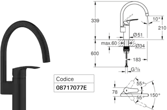
Eurosmart | bocca alta
