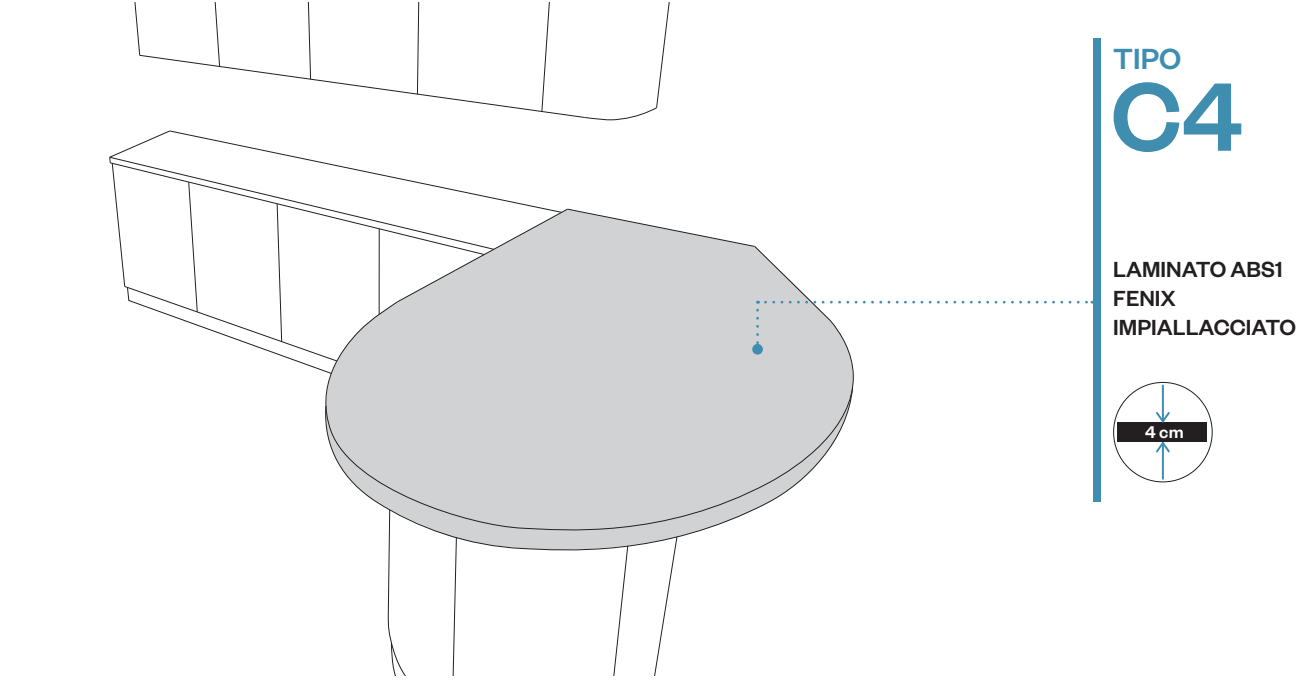
Penisola sagomata “C4”. Disponibile nello spessore 4 cm. Da realizzare solo con gambone di sostegno e in appoggio su basi.
