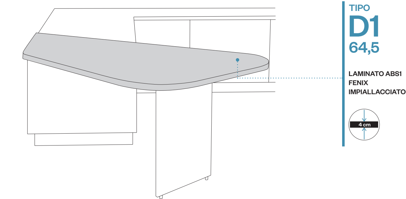
Penisola sagomata “D1” 64,5 con 2 angoli stondati. Disponibile nello spessore 4 cm. Da realizzare in appoggio su basi o ancorata a parete mediante l’apposita piastra.
