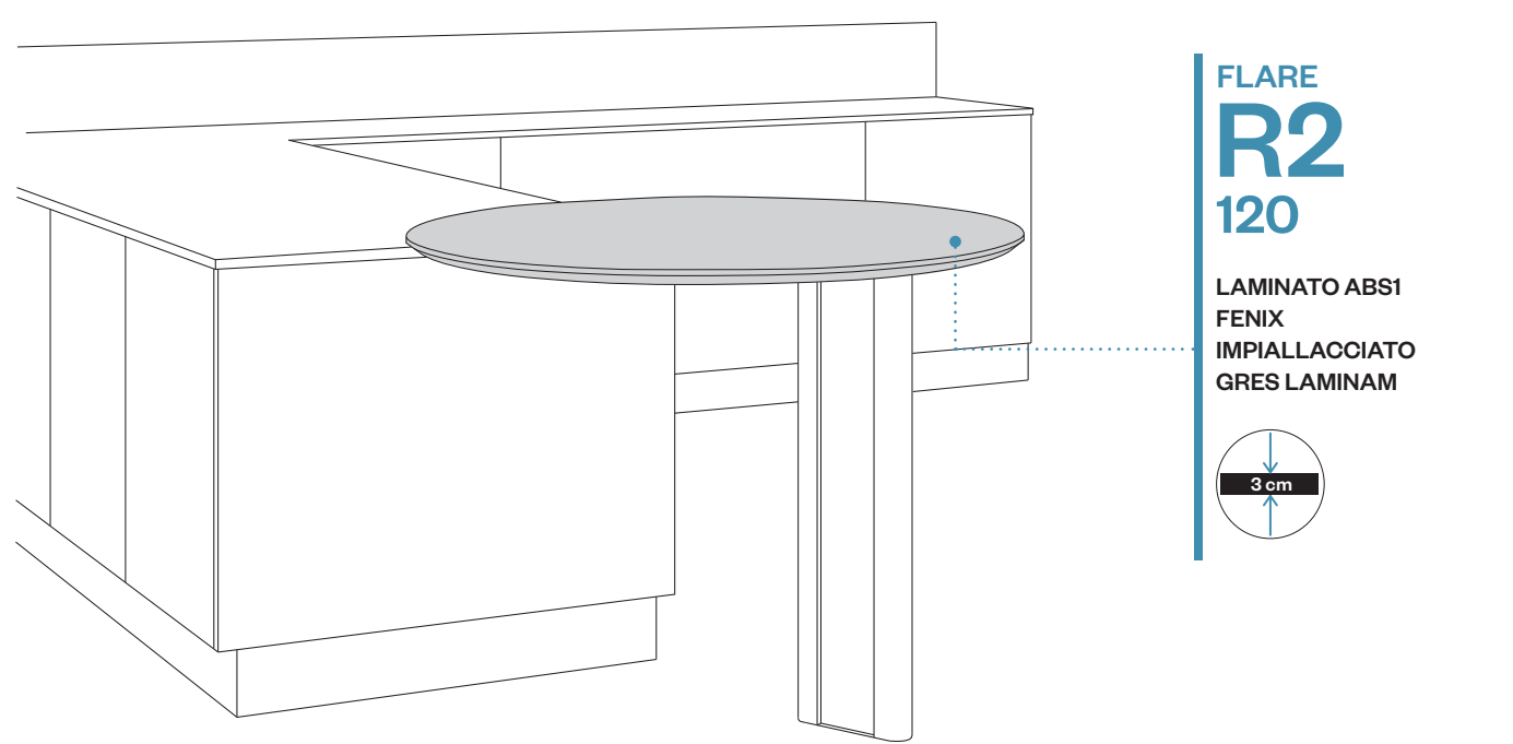
Penisola rotonda “R2” con profilo inclinato. Disponibile nello spessore 3 cm. Da realizzare solo con gambone di sostegno e in appoggio su basi.
