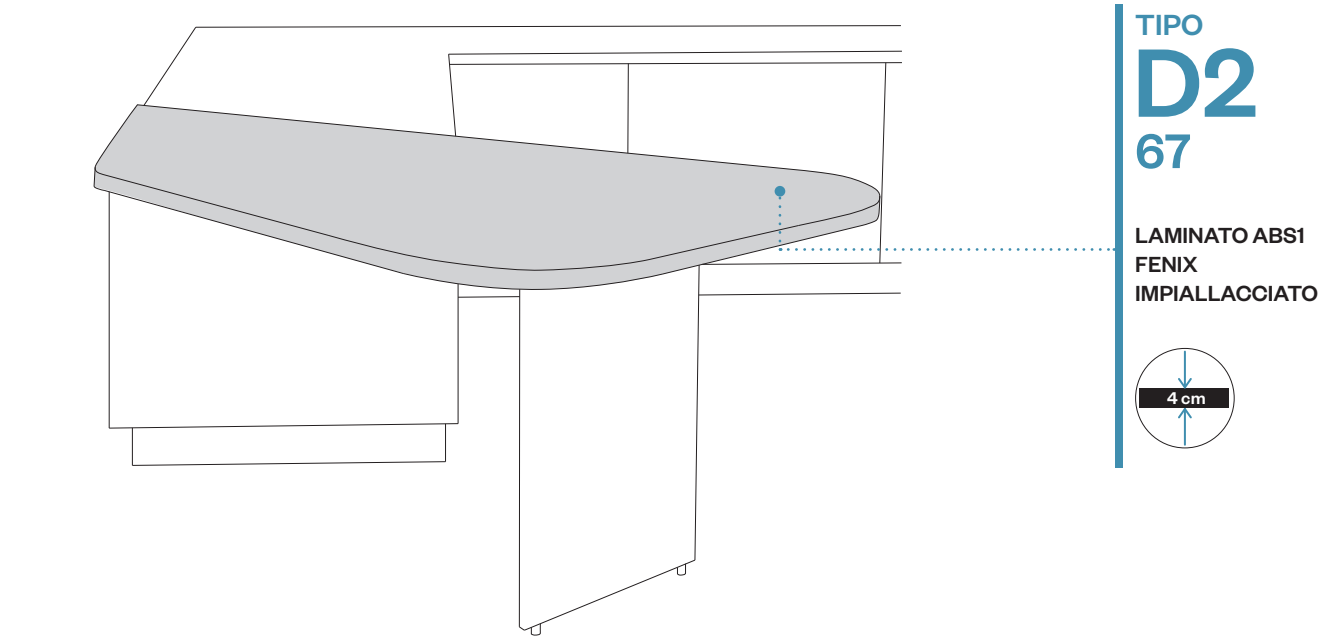
Penisola sagomata “D2” 67 con 2 angoli stondati. Disponibile nello spessore 4 cm. Da realizzare in appoggio su basi o ancorata a parete mediante l’apposita piastra.
