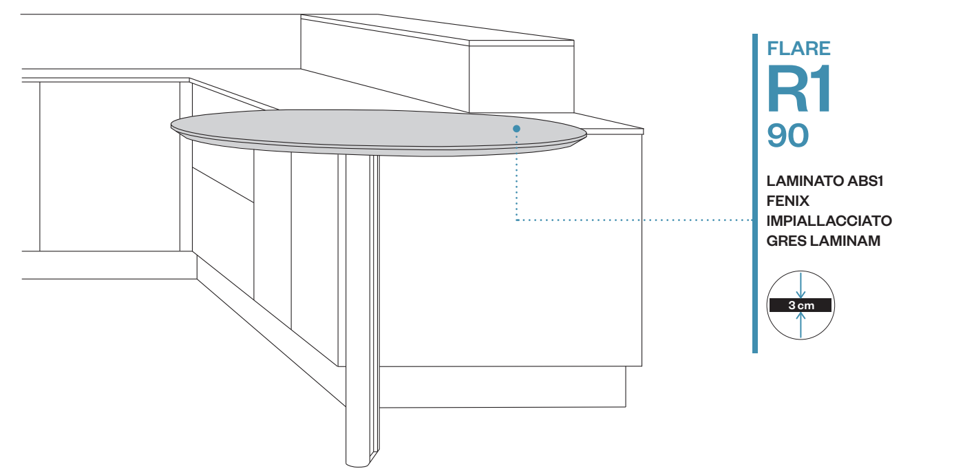
Penisola rotonda “R1” con profilo inclinato. Disponibile nello spessore 3 cm. Da realizzare solo con gambone di sostegno e in appoggio su basi.
