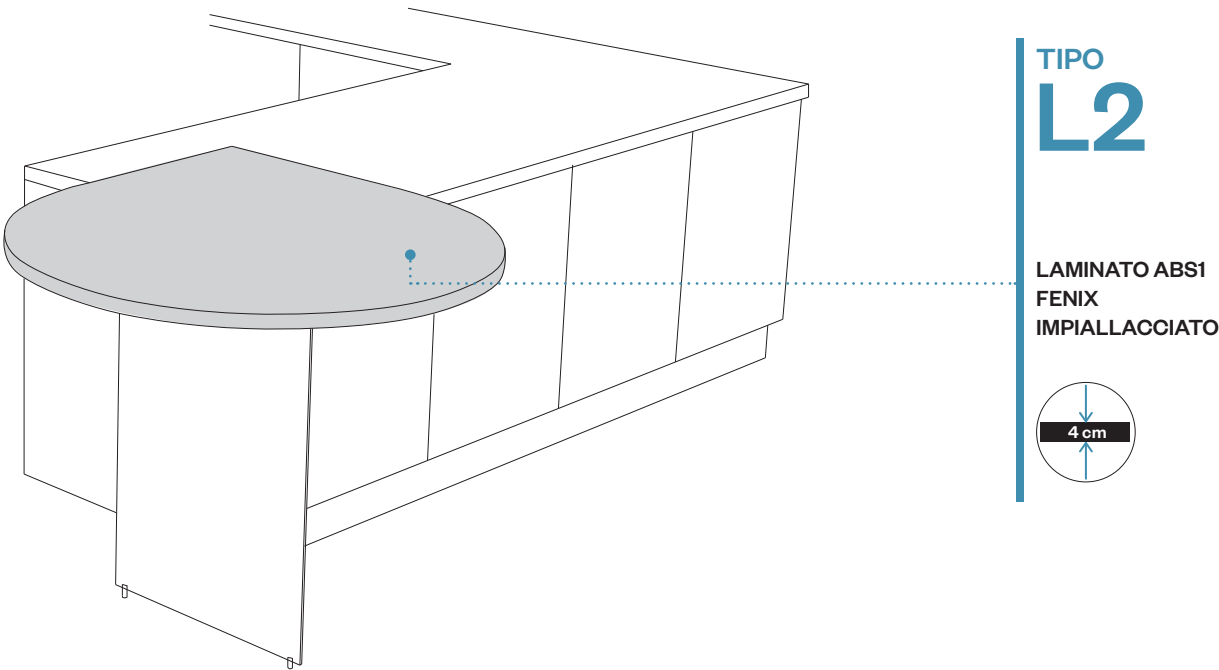
Penisola sagomata “L2” a goccia. Disponibile nello spessore 4 cm. Da realizzare in appoggio su basi o ancorata a parete mediante l'apposita piastra.
