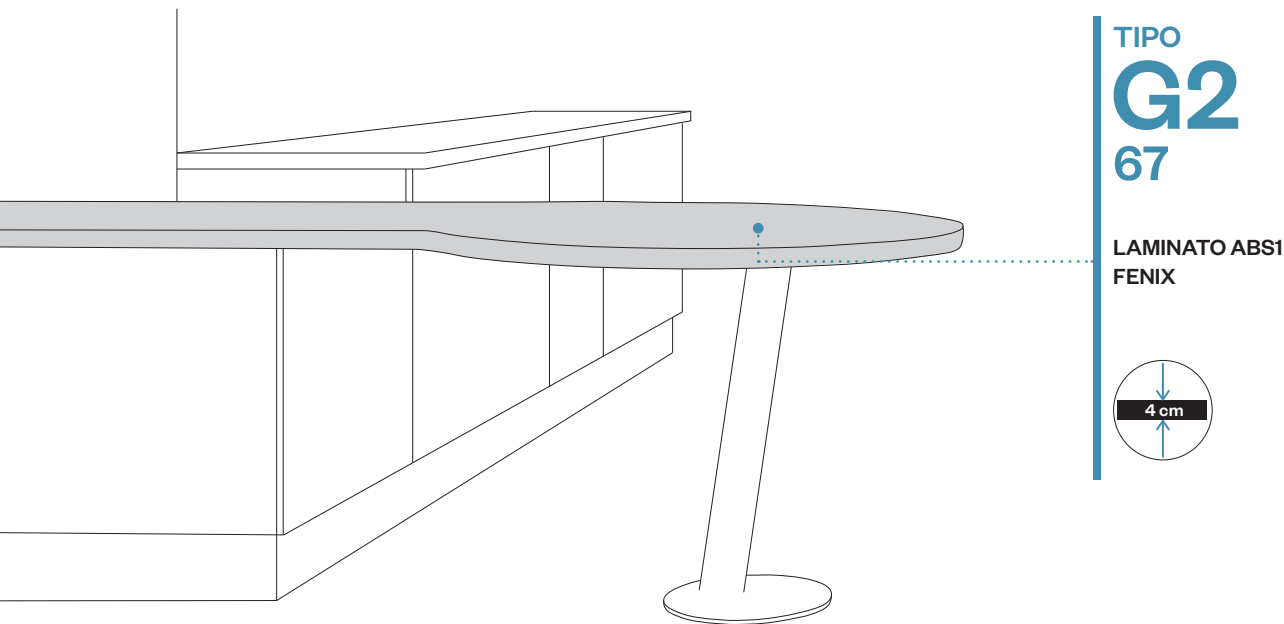
Penisola sagomata “G2” 67 a goccia. Disponibile nello spessore 4 cm. Da realizzare in appoggio su basi o ancorata a parete mediante l’apposita piastra.
