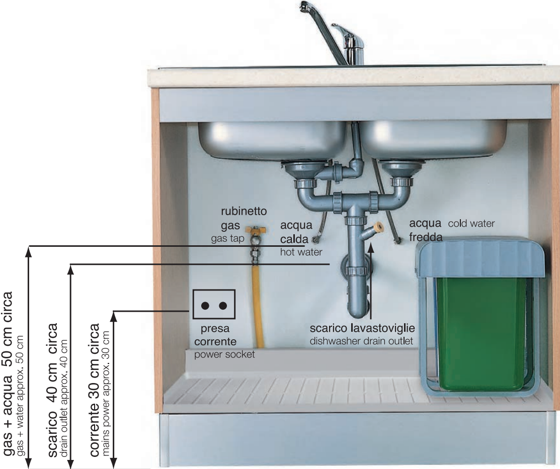
SOTTOLAVELLO CON ANTE SINK BASE UNIT WITH DOORS
