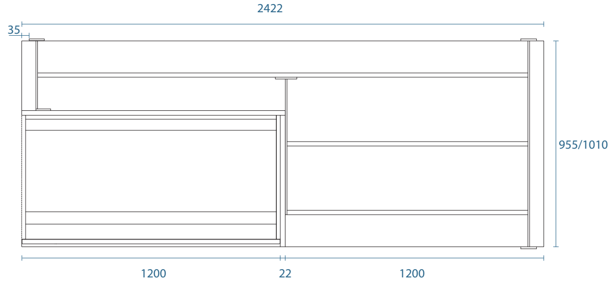
ESEMPIO DI COMPOSIZIONE ISOLA CON BASI E TOP A SBALZO 120 CM EXAMPLE OF ISLAND COMPOSITION WITH BASE UNITS AND OVERHANF WORKTOP 120 CM EXEMPLE DE COMPOSITION D'UN ÎLOT AVEC DES ÉLÉMENTS BAS ET UN PDT EN PORTE-À-FAUX DE 120 CM EJEMPLO DE COMPOSICIÓN DE ISLA CON MUEBLES BAJOS Y ENCIMERA VOLADIZA DE 120 CM ПРИМЕР ОСТРОВНОЙ КОМПОЗИЦИИ С БАЗОВЫМИ ШКАФАМИ И КОНСОЛЬНОЙ СТОЛЕШНИЦЕЙ 120 CM
