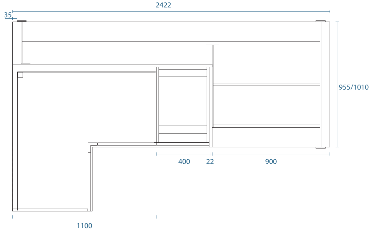
ESEMPIO DI COMPOSIZIONE PENISOLA CON BASE ANGOLO E TOP A SBALZO 90 CM EXAMPLE OF PENINSULA COMPOSITION WITH CORNER BASE UNIT AND OVERHANF WORKTOP 90 CM EXEMPLE DE COMPOSITION DE PÉNINSULE AVEC BASE D'ANGLE ET UN PDT EN PORTE-À-FAUX DE 90 CM EJEMPLO DE COMPOSICIÓN DE PENÍNSULA CON BASE ESQUINERA Y ENCIMERA VOLADIZA DE 90 CM ПРИМЕР КОМПОЗИЦИИ ПОЛУОСТРОВА С УГЛОВЫМ ОСНОВАНИЕМ И КОНСОЛЬНОЙ СТОЛЕШНИЦЕЙ 90 CM
