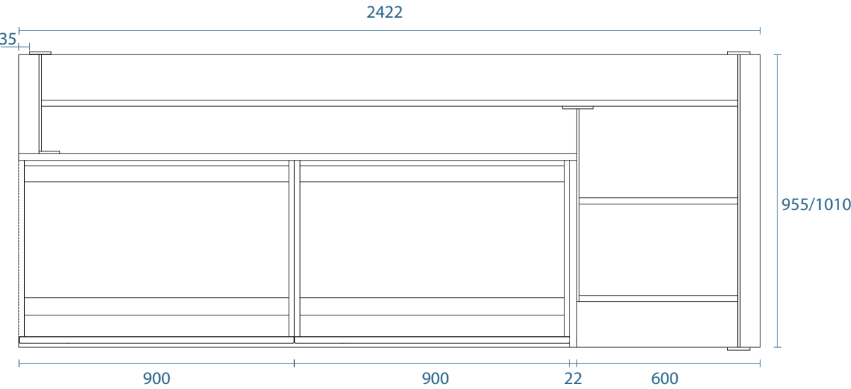
ESEMPIO DI COMPOSIZIONE ISOLA CON BASI E TOP A SBALZO 60 CM EXAMPLE OF ISLAND COMPOSITION WITH BASE UNITS AND OVERHANF WORKTOP 60 CM EXEMPLE DE COMPOSITION D'UN ÎLOT AVEC DES ÉLÉMENTS BAS ET UN PDT EN PORTE-À-FAUX DE 60 CM EJEMPLO DE COMPOSICIÓN DE ISLA CON MUEBLES BAJOS Y ENCIMERA VOLADIZA DE 60 CM ПРИМЕР ОСТРОВНОЙ КОМПОЗИЦИИ С БАЗОВЫМИ ШКАФАМИ И КОНСОЛЬНОЙ СТОЛЕШНИЦЕЙ 60 CM
