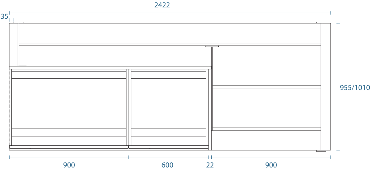
ESEMPIO DI COMPOSIZIONE ISOLA CON BASI E TOP A SBALZO 90 CM EXAMPLE OF ISLAND COMPOSITION WITH BASE UNITS AND OVERHANF WORKTOP 90 CM EXEMPLE DE COMPOSITION D'UN ÎLOT AVEC DES ÉLÉMENTS BAS ET UN PDT EN PORTE-À-FAUX DE 90 CM EJEMPLO DE COMPOSICIÓN DE ISLA CON MUEBLES BAJOS Y ENCIMERA VOLADIZA DE 90 CM ПРИМЕР ОСТРОВНОЙ КОМПОЗИЦИИ С БАЗОВЫМИ ШКАФАМИ И КОНСОЛЬНОЙ СТОЛЕШНИЦЕЙ 90 CM
