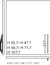
PENSILE WALL UNIT
