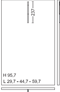
COLONNA ANTA CESTELLO ESTRAIBILE COLUMN PULL-OUT BASKET DRAWER DOOR
