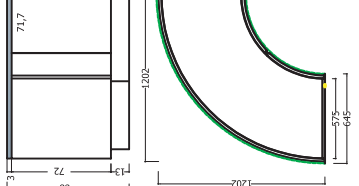
ISOLA CIRCOLARE TIPO "D" 1202 X 1224 ROUND ISLAND UNIT TYPE "D"
