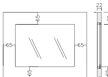
anta vetro con presa maniglia tipo "B" glass door with type "B" handle grip
