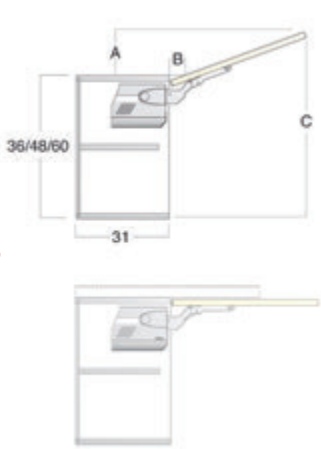
SCHEMA MONTAGGIO LIMITATORE PER RIBALTA H 36 FLAP DOOR LIMITER INSTALLATION DIAGRAM H 36
