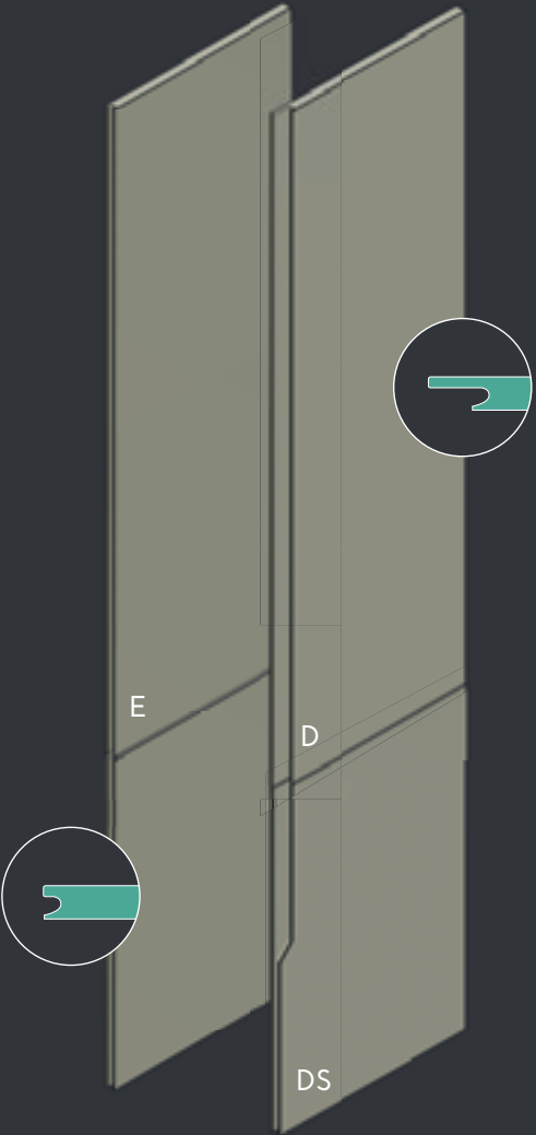
TIPO D - DS - E ANTE PER COLONNE CON PRESA VERTICALE CON E SENZA SAGOMATURA
