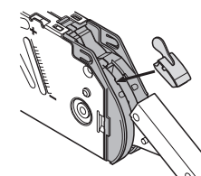
SCHEMA MONTAGGIO LIMITATORE LIMITER INSTALLATION DIAGRAM
